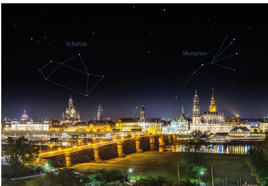
(7) Sterne über Dresden – Anfang August 22 Uhr. Altstadtpanorama mit Augustusbrücke und Elbe. Am Himmel stehen Schütze und Skorpion.
