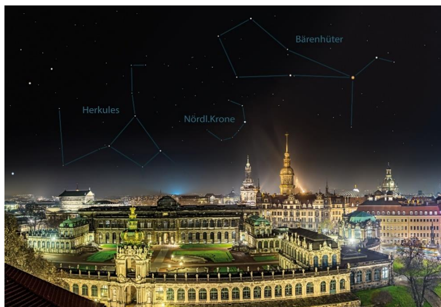
(8) Sterne über Dresden – Mitte März 22 Uhr. Blick über den Zwinger mit dem Kronentor links. Oben Herkules, Nördliche Krone und Bärenhüter.
