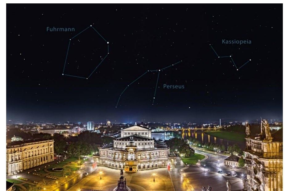
(9) Sterne über Dresden – Mitte Mai 22 Uhr. Zwinger, Semperoper, Elbe, Hofkirche. Mit Fuhrmann, Perseus und Kassiopeia.
