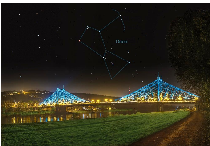
(10) Sterne über Dresden – Mitte Dezember 20 Uhr. Das Blaue Wunder – historische Hängebrücke. Darüber thront der Himmelsjäger Orion.
