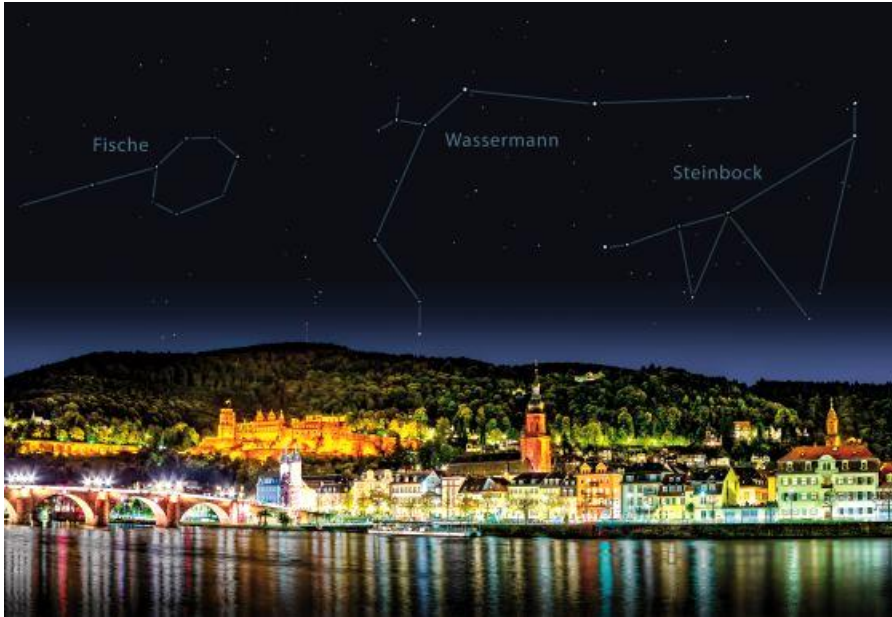
(4) Sterne über Heidelberg – Mitte Sept. 22 Uhr. Über den Neckar zur Altstadt, links das Schloss. Darüber Fische, Wassermann und Steinbock.
